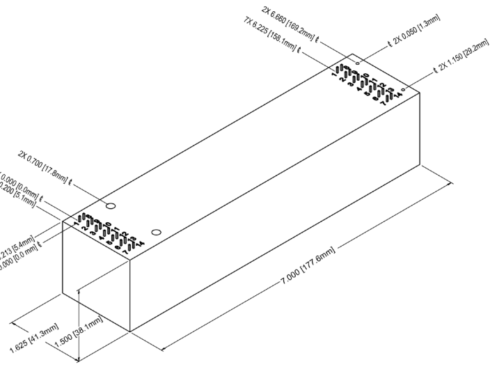
30EFL Module
