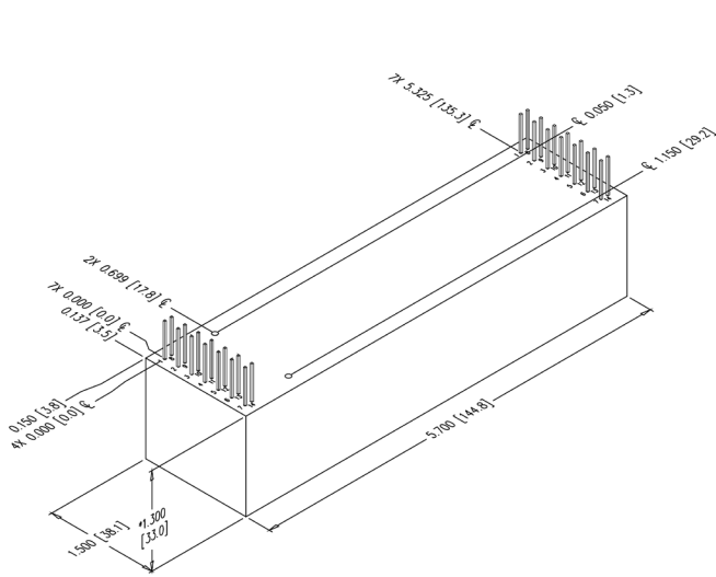
15EFL Module
